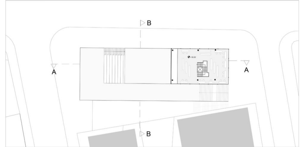
1/200 +16.00 Kot Planı
