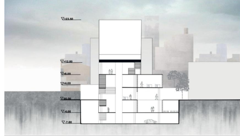
1/200 AA' Kesiti
