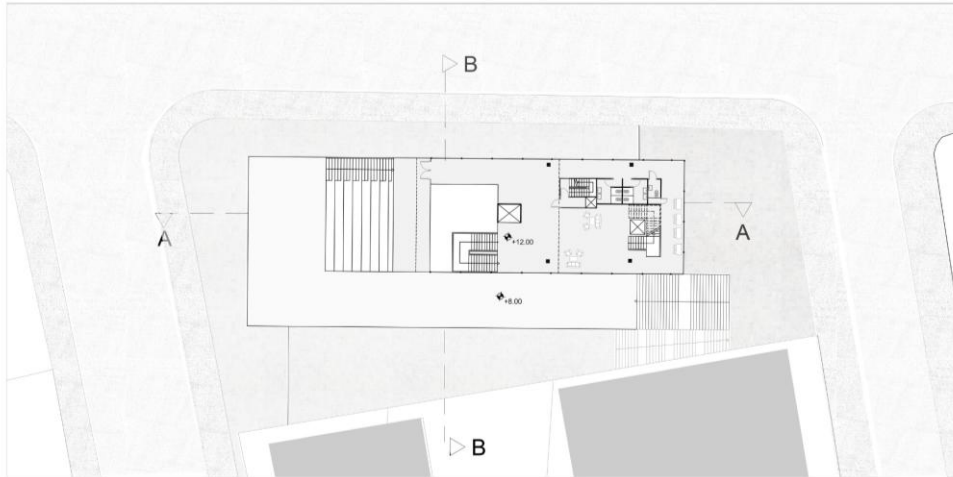
1/200 +12.00 Kot Planı
